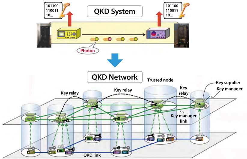
[그림 1] 양자암호키 분배 시스템과 분배망의 개념
