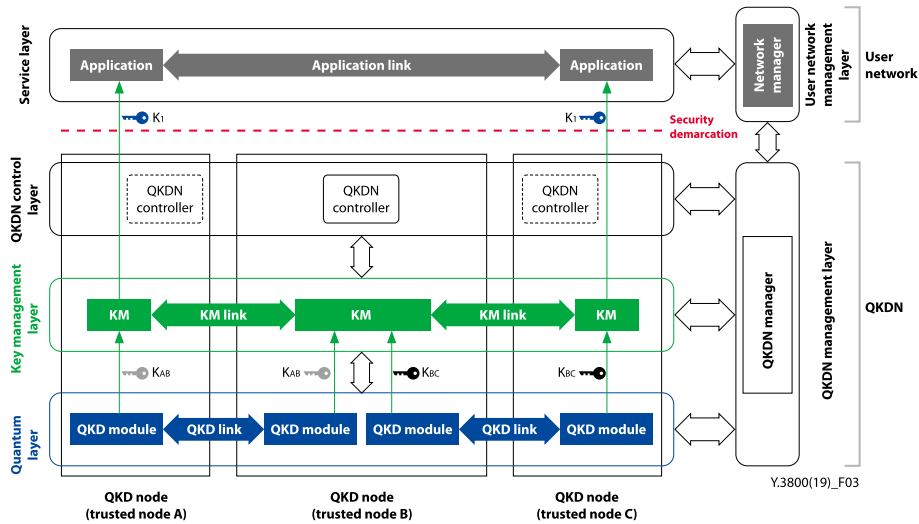
[그림 3] 양자암호키 분배망과 사용자 망의 개념적 구조
