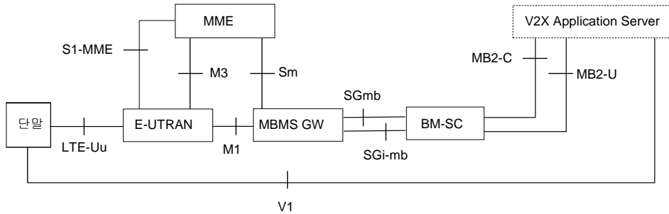
(그림 5) MBMS 기반 V2X 서비스를 위한 네트워크 아키텍처 참조 모델 (MB2 사용)
