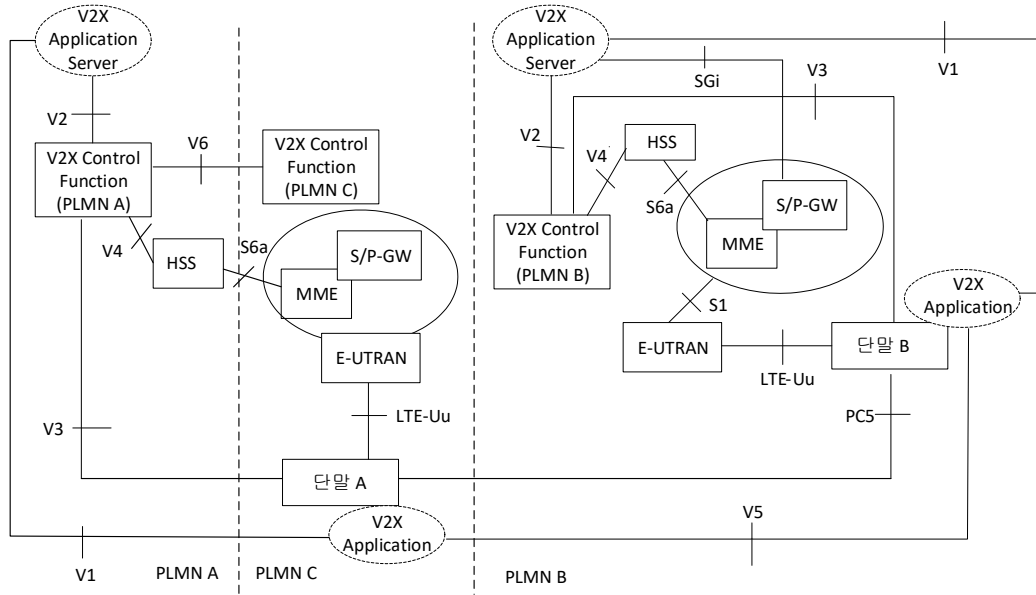
(그림 4) PC5/Uu inter-PLMN V2X 서비스를 위한 네트워크 아키텍처 참조 모델
