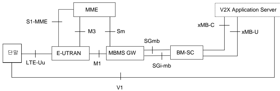
(그림 6) MBMS 기반 V2X 서비스를 위한 네트워크 아키텍처 참조 모델 (xMB 사용)
