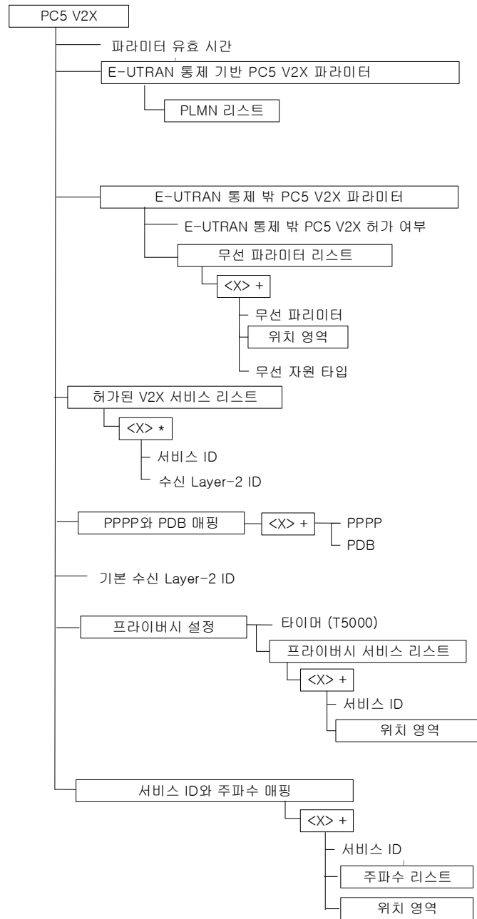
(그림 8) PC5 V2X OMA-DM 관리 객체
