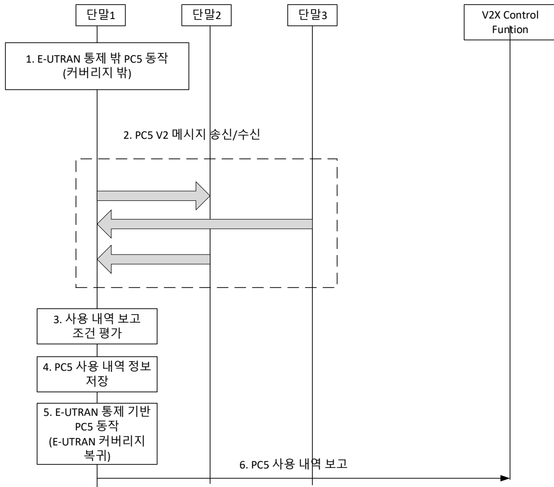
(그림 10) Off-line 과금 정보 보고
