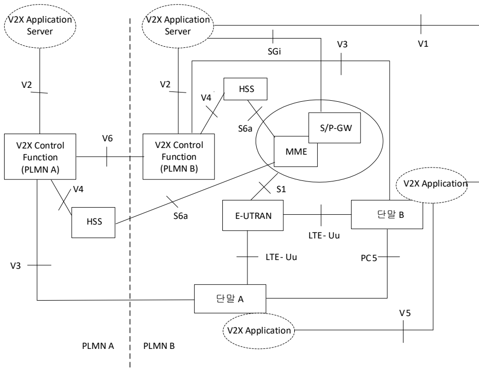
(그림 3) PC5/Uu V2X 로밍 서비스를 위한 네트워크 아키텍처 참조 모델
