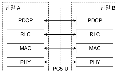
(그림 1) 사이드링크 (Sidelink) 통신을 위한 사용자 평면 프로토콜 스택
